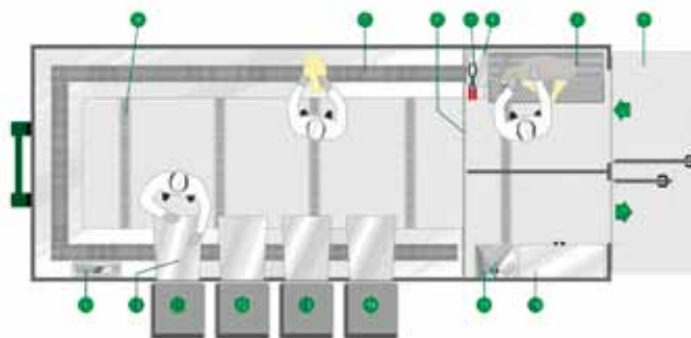
Станция уоя для овец и коз М5-М7
